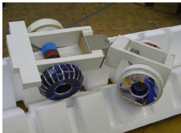
Рисунок 2-Конструкция сочленённых рам с шарнирным соединением (материал: тонкий и гофрированный картон, пенопласт, пластиковые крышки, проволока, жёсть)
